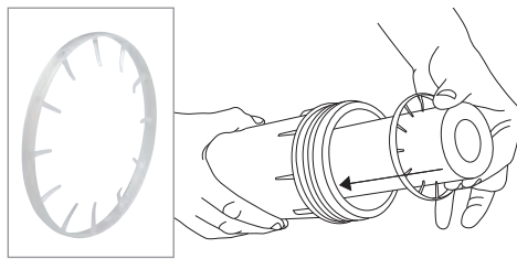
FILTERFIT Cartridge centering device 滤芯中心定位装置
